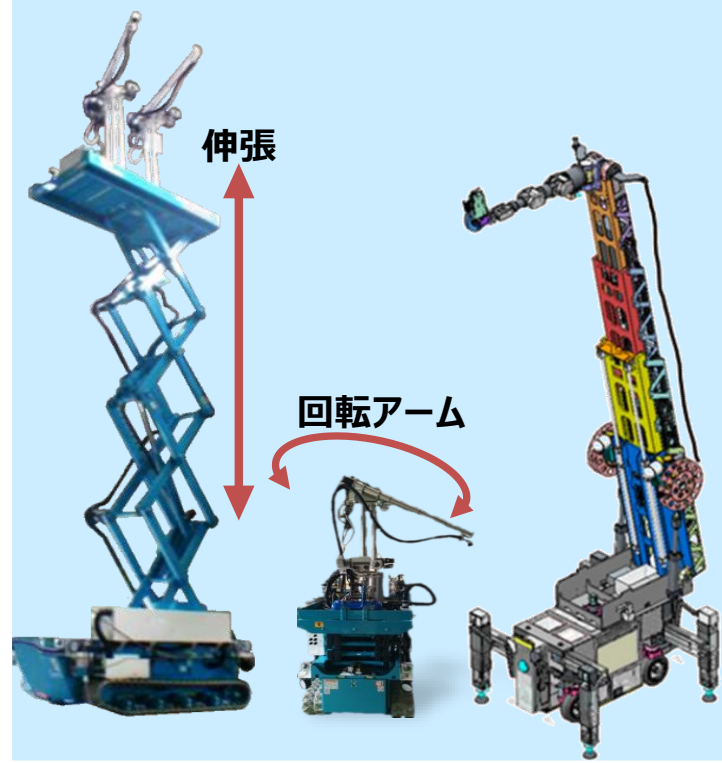
高圧水噴射
