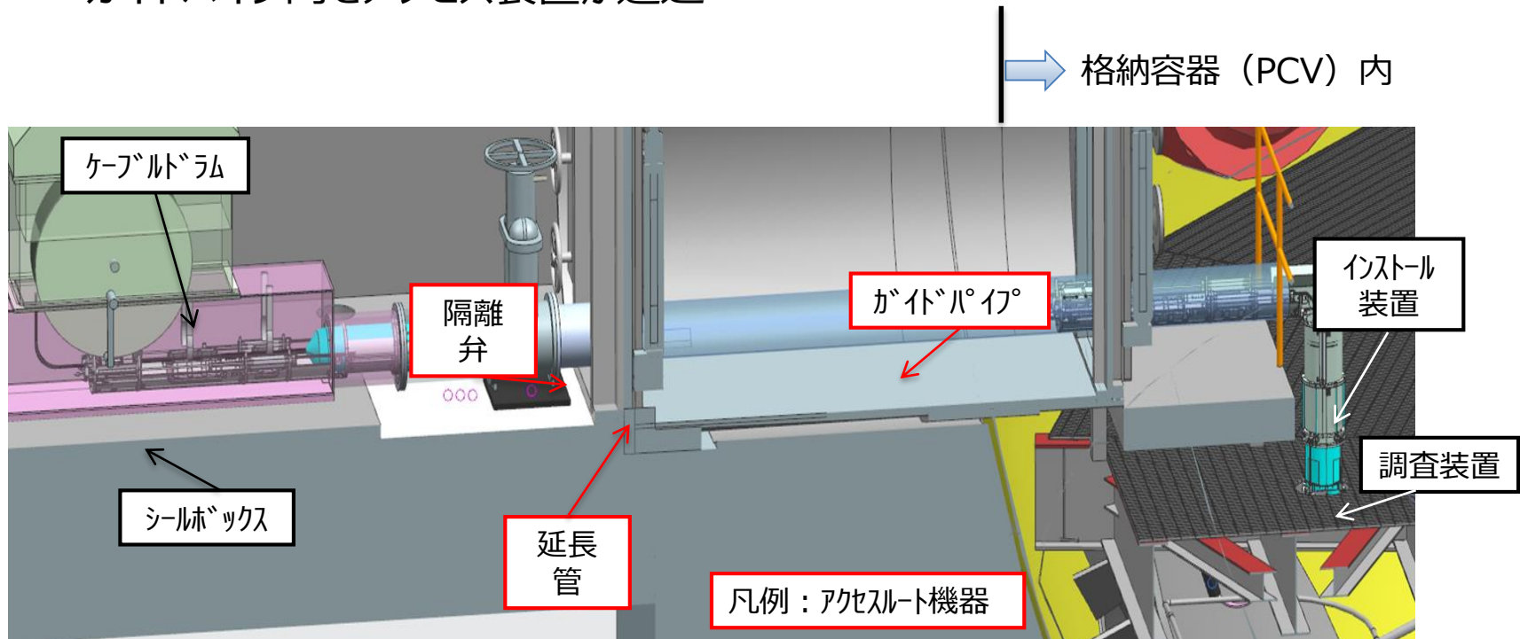
格納容器（PCV）バウンダリの構成(案)
