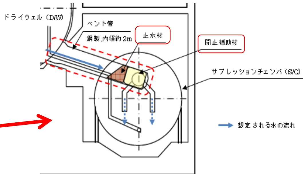
PCV下部補修の対象範囲
